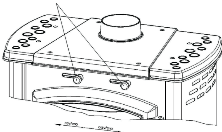
Rukojeť regulátoru sekundárního vzduchu
